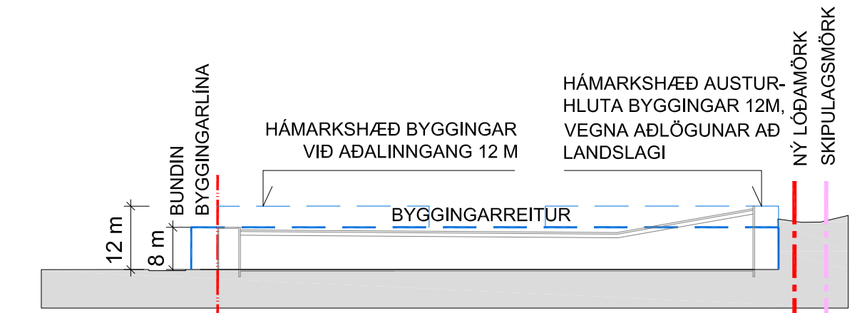
KENNISNEIDING R2 KAUPTÚN 3 GILDANDI SKIPULAG A1) 1:1000
