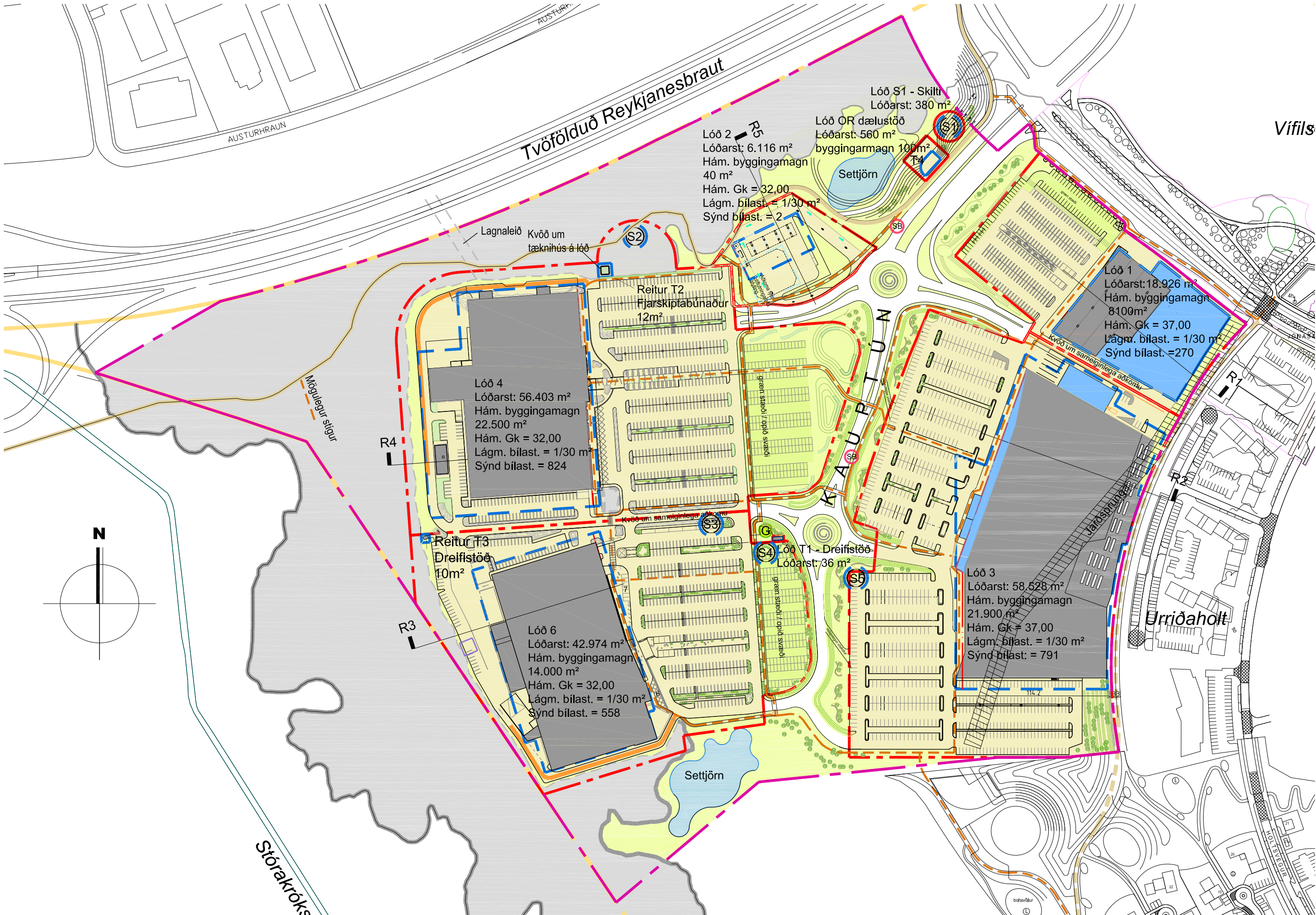
Tillaga að breyttu deiliskipulagi
