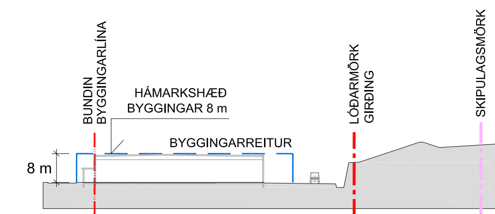
KENNISNEIDING R1 KAUPTÚN 1 GILDANDI SKIPULAG A1) 1:1000
