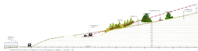
Mynd 5. Frágangur við Ásvallabraut til að draga úr hávaða frá umferð - Mön, girðing og gróður við Furuás.
