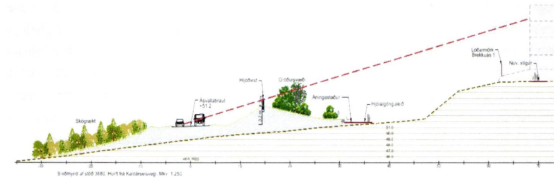
Mynd 4. Frágangur við Ásvallabraut til að draga úr hávaða frá umferð-Mön, girðing og gróður við Brekkuás.
