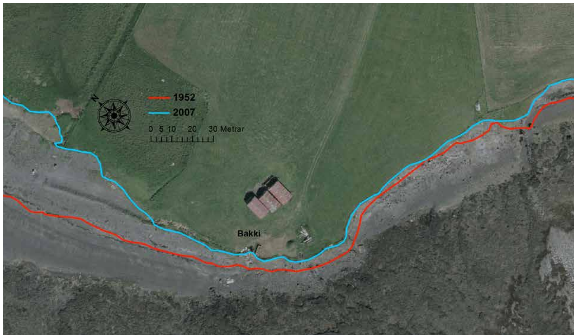
Mynd 4.1.16 Sýnilegar breytingar á strandlínu frá 1952 - 2007
