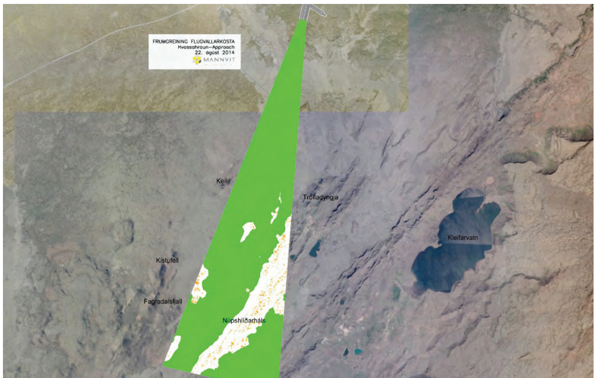
Mynd 23 Hvassahraun – 15 km hindrunarflötur, nákvæmnisaðflug á aðalflugbraut (hvítar hæðarlínur sýna land sem nær upp í flötinn)
