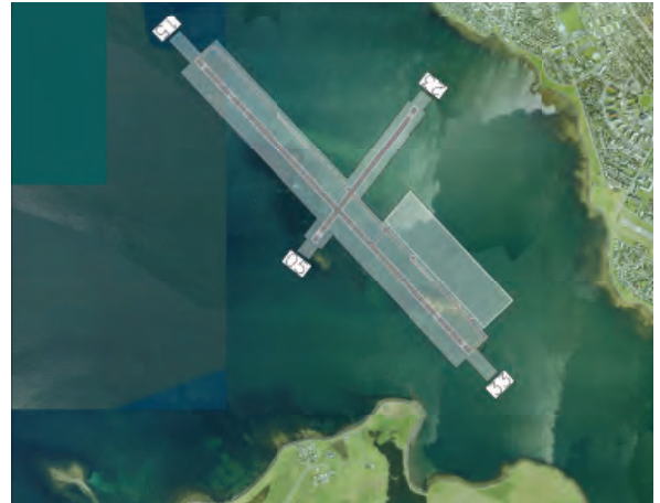
Mynd 32 Lögusker - alhliða innanlandsflugvöllur með 3.000 m aðalflugbraut og auknu athafnasvæði
