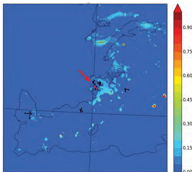
Mynd 7 Hlutfall mikillar ókyrrðar fyrir aðflug á braut 15/33 á Bessastaðanesi
