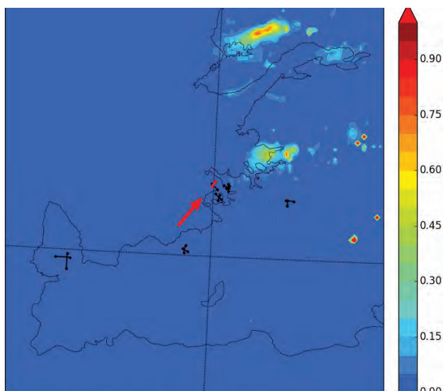
Mynd 34 Hlutfall mikillar ókyrrðar fyrir aðflug á braut 05/23 á Lönguskerjum
