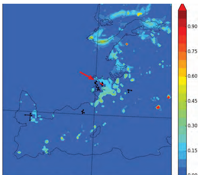
Mynd 43 Hlutfall mikillar ókyrrðar fyrir aðflug á braut 13/31 í Vatnsmýri
