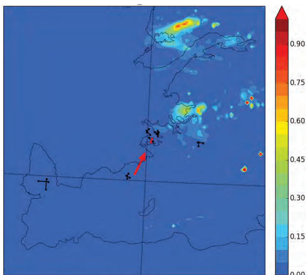
Mynd 6 Hlutfall mikillar ókyrrðar fyrir aðflug á braut 03/21 á Bessastaðanesi
