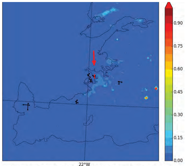
Mynd 42 Hlutfall mikillar ókyrrðar fyrir aðflug á braut 01/19 í Vatnsmýri
