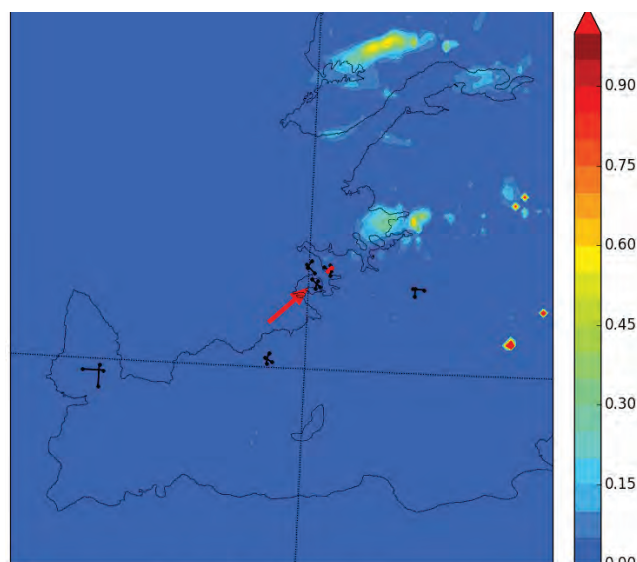
Mynd 44 Hlutfall mikillar ókyrrðar fyrir aðflug á braut 06/24 í Vatnsmýri
