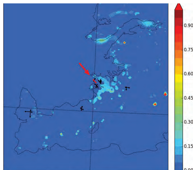
Mynd 35 Hlutfall mikillar ókyrrðar fyrir aðflug á braut 15/33 á Lönguskerjum
