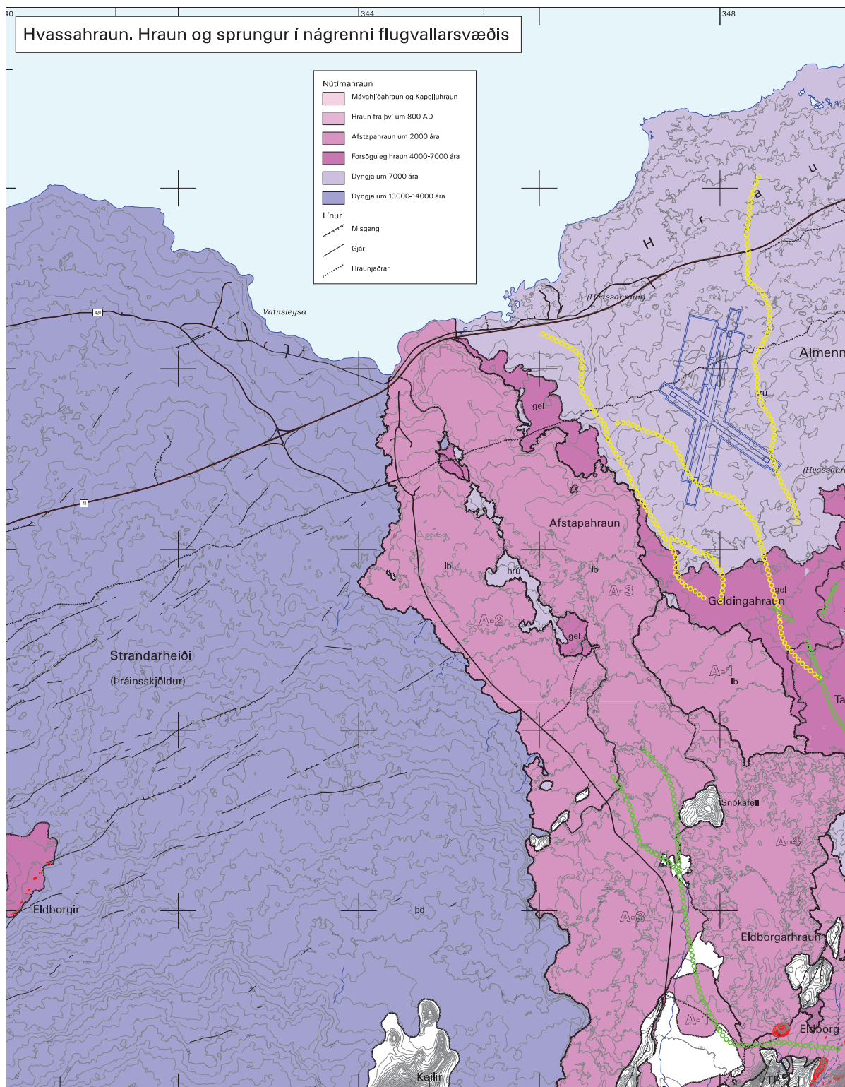
Mynd 29 Hvassahraun – hraun og sprungur í nágrenni flugvallarstæðis
