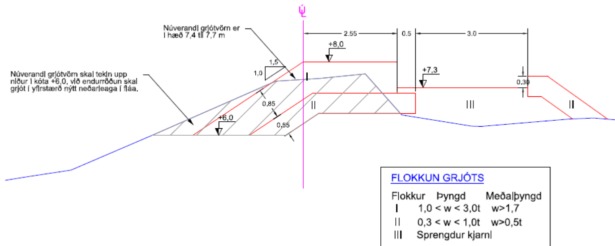
Mynd 1 Snið í sjónvörn, hækkun upp í kóta +8,0
