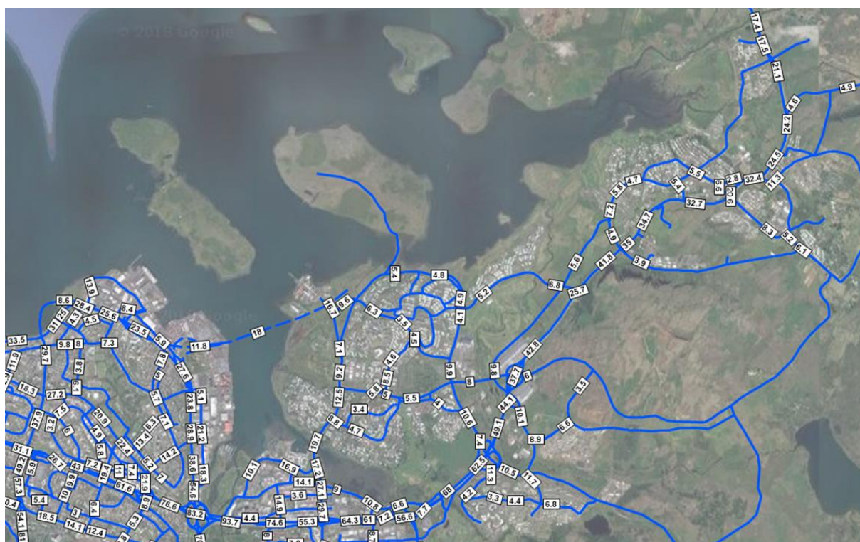
Mynd 5.4 Niðurstaða spár 2030 fyrir Sundabraut í göngum, áfangi 1. Í Ártúnsbrekku er umferð rúmlega 94. 000 bílar á sólarhring (HVDU) og yfir Gulllinbrú fara tæplega 20.000 bílar (HVDU). Umferð á Vesturlandsvegi í Mosfellsbæ er í kringum 33.000 bílar (HVDU)
