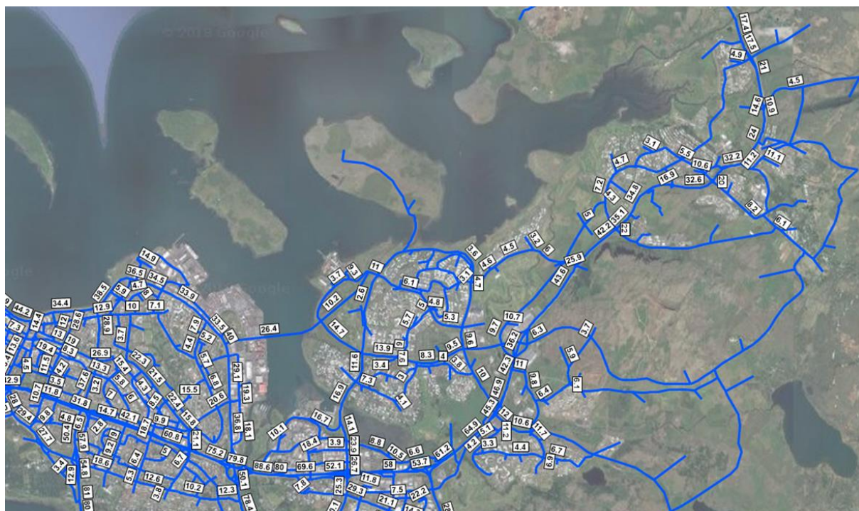
Mynd 5.3 Niðurstaða spár 2030 fyrir Sundabraut með brú, áfangi 1. Í Ártúnsbrekku er umferð tæplega 89.000 bílar á sólarhring (HVDU) og yfir Gulllinbrú fara tæplega 17.000 bílar (HVDU). Umferð á Vesturlandsvegi í Mosfellsbæ er í kringum 33.000 bílar (HVDU)
