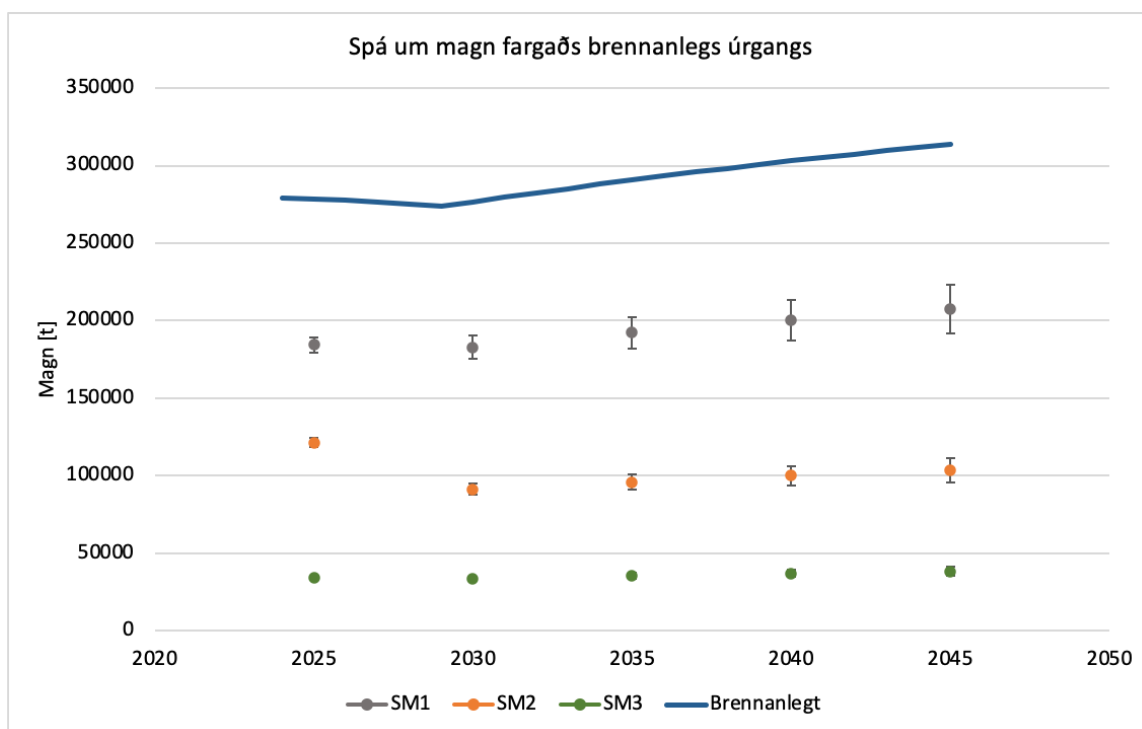
Mynd 19. Spá um þörf fyrir förgun brennanlegs úrgangs á Íslandi árin 2025 til 2045. Öryggisbilið gefur til kynna óvissu byggða á mannfjöldaspá Hagstofu Íslands.
