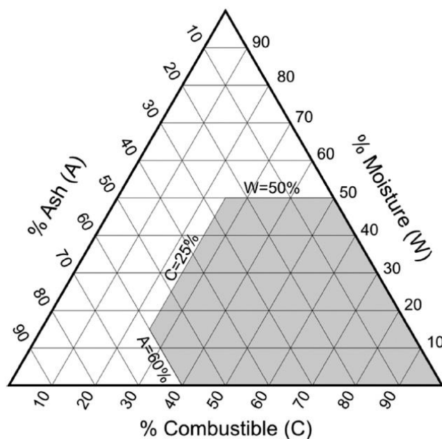
Mynd 1. Teikning Tanners. Úrgangur sem fellur innan við grúa svæðið er hægt að brenna án eldsneytisaðstoðar (Christensen, 2011).
