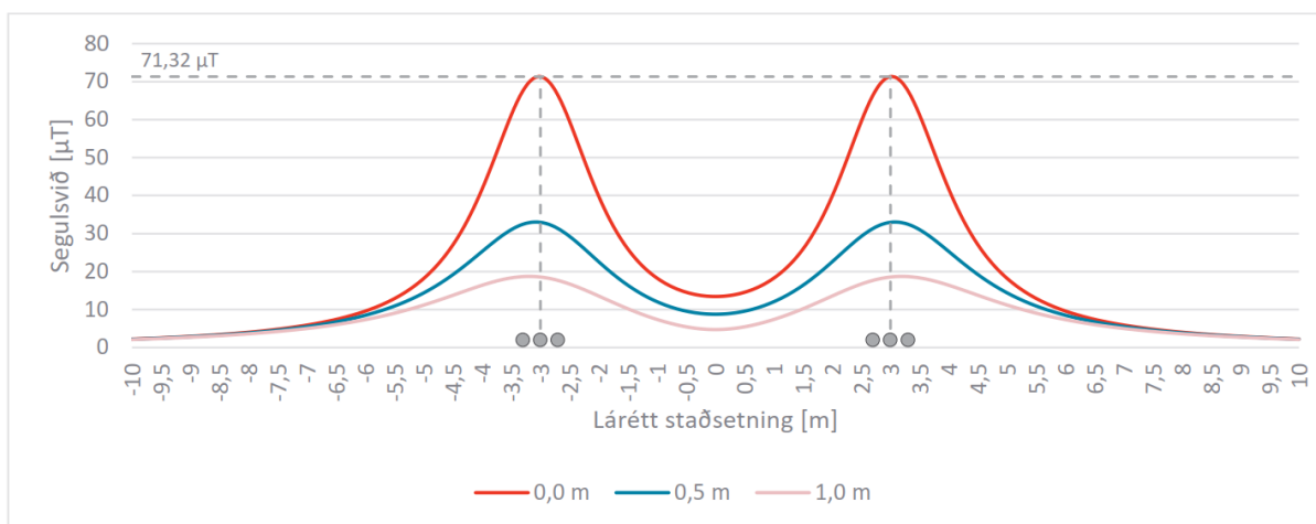
Mynd 4.10 Segulsvið frá mögulegum 220 kV jarðstreng þar sem 6 m eru á milli strengsetta. Viðmiðunargildi ICNIRP, 200 \mu\text{T} er það hátt að það er ekki sýnt á línuritinu.
