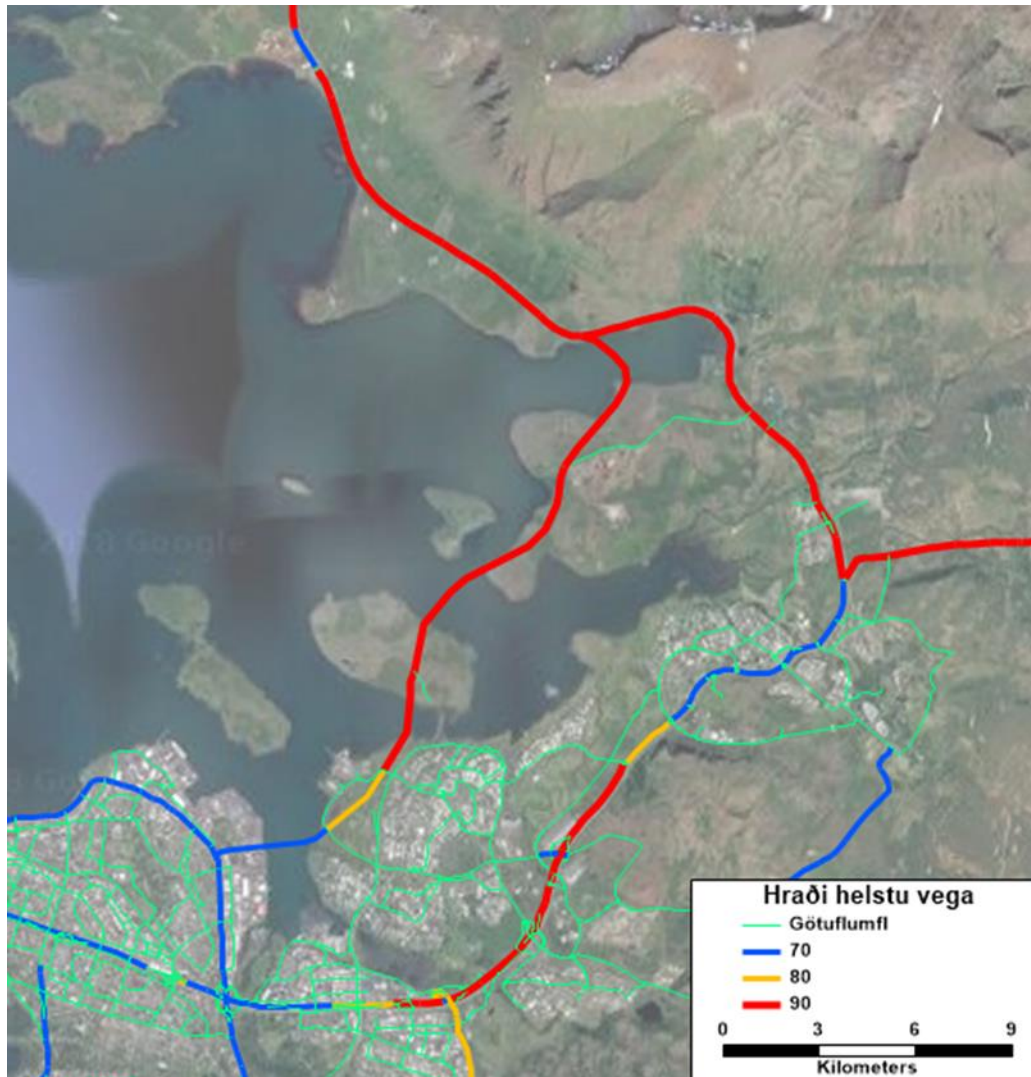
Mynd 3.4 Hraði um helstu vegi m.v. tilfelli Sundabrautar á brú. Hér er miðað við áætlaðan hraði í frjálsu flæði og þarf hann ekki í öllum tilfellum að vera merktur hámarkshraði.
