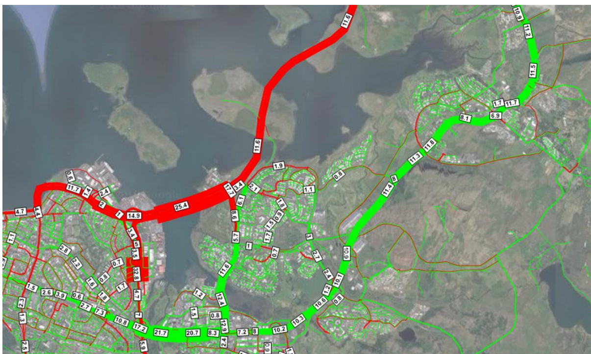
Mynd 5.12 Mismunakort fyrir spá 2030. Myndin sýnir hvar umferð eykst eða minnkar við tilkomu Sundabrautar með brú samanborið við 0-tilfellið (engin Sundabraut), þar sem rauðir vegbútar sýna hvar umferð eykst. Sjá má að umferð í gegnum Mosfellsbæ minnkar um u.þ.b. 12.000 bíla (HVDU)
