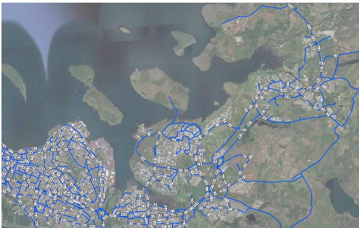
Mynd 5.2 Niðurstaða spár fyrir 2030 í tilfelli 0-kostar. Í Ártúnsbrekku er umferð rúmlega 110.000 bílar á sólarhring (HVDU) og yfir Gullinbrú fara rúmlega 32.000 bílar (HVDU). Umferð á Vesturlandsvegi í Mosfellsbæ er í kringum 33.000 bílar (HVDU)
