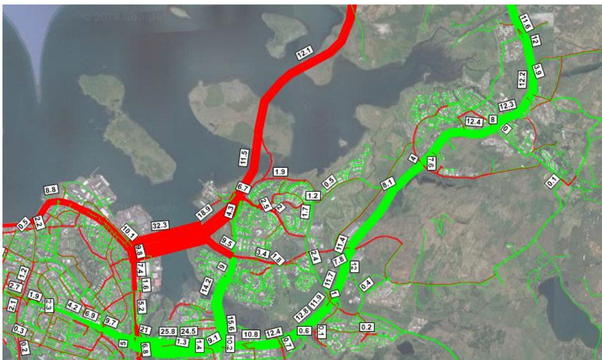
Mynd 5.11 Mismunakort fyrir spá 2030. Myndin sýnir hvar umferð eykst eða minnkar við tilkomu Sundabrautar með brú samanborið við 0-tilfellið (engin Sundabraut), þar sem rauðir vegbútar sýna hvar umferð eykst. Sjá má að umferð í gegnum Mosfellsbæ minnkar um u.þ.b. 12.000 bíla (HVDU)
