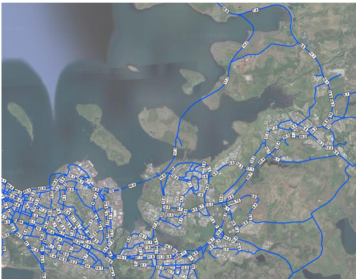
Mynd 5.14 Niðurstaða spár 2050+ fyrir Sundabraut í göngum. Í Ártúnsbrekku er umferð um 110.000 bílar á sólarhring (HVDU) og yfir Gulllinbrú fara um 28.000 bílar (HVDU). Umferð á Vesturlandsvegi í Mosfellsbæ er í kringum 30.000 bílar (HVDU)
