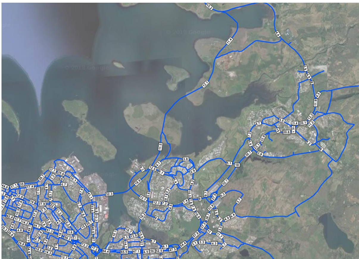
Mynd 5.5 Niðurstaða spár 2030 fyrir Sundabraut með brú. Í Ártúnsbrekku er umferð tæplega 85. 000 bílar á sólarhring (HVDU) og yfir Gullinbrú fara rúmlega 18.000 bílar (HVDU). Umferð á Vesturlandsvegi í Mosfellsbæ er í kringum 20.000 bílar (HVDU)
