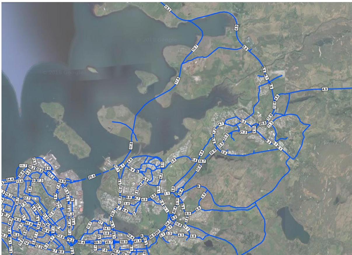
Mynd 5.7 Niðurstaða spár 2030 fyrir Sundabraut í göngum. Í Ártúnsbrekku er umferð tæplega 85.000 bílar á sólarhring (HVDU) og yfir Gullinbrú fara rúmlega 20.000 bílar (HVDU). Umferð á Vesturlandsvegi í Mosfellsbæ er í kringum 20.000 bílar (HVDU).
