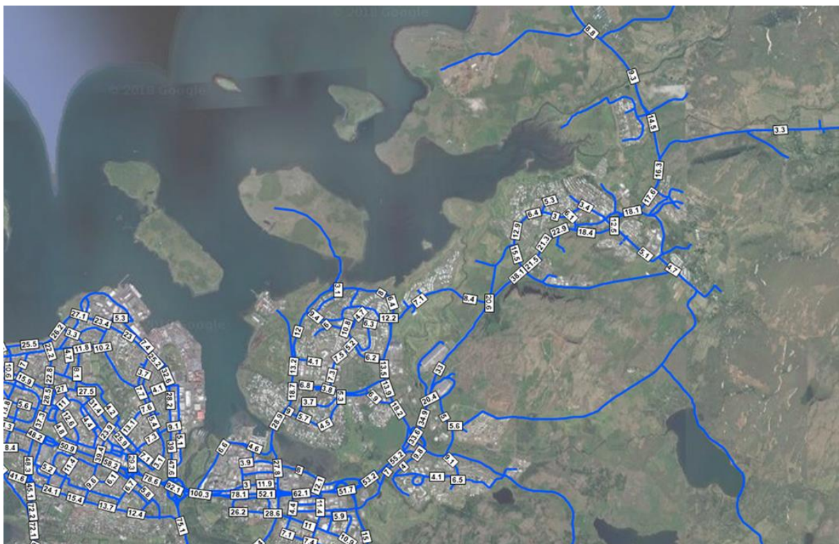
Mynd 5.1 Grunnár 2016. Í Ártúnsbrekku eru rétt rúmlega 100 þúsund bílar á sólarhring (HVDU) og yfir Gullinbrú fara tæplega 29.000 bílar (HVDU). Umferð á Vesturlandsvegi í Mosfellsbæ er rétt um 18.500 bílar (HVDU)
