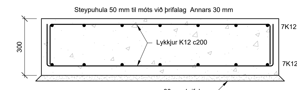
f SNIÐ 1:10
