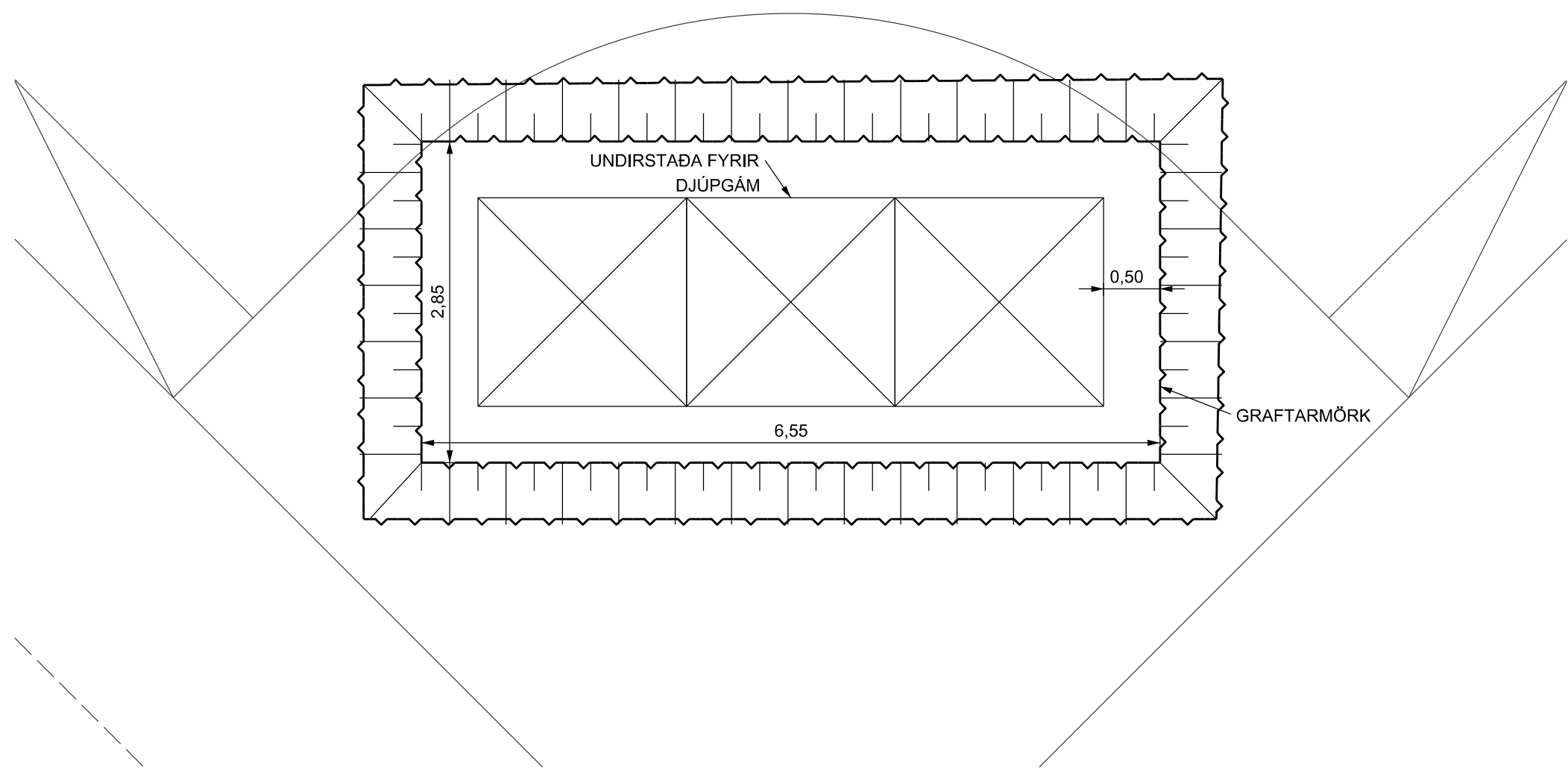
PLANMYND - DJÚPGÁMAR
