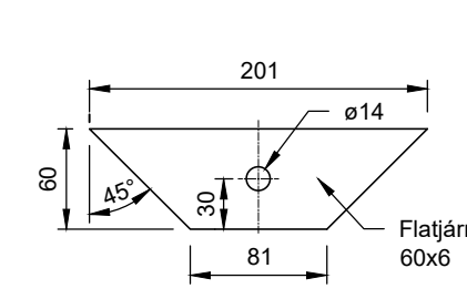
P1 PLATA 1 1:4
