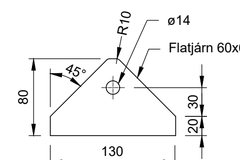
P2 PLATA 2 1:4
