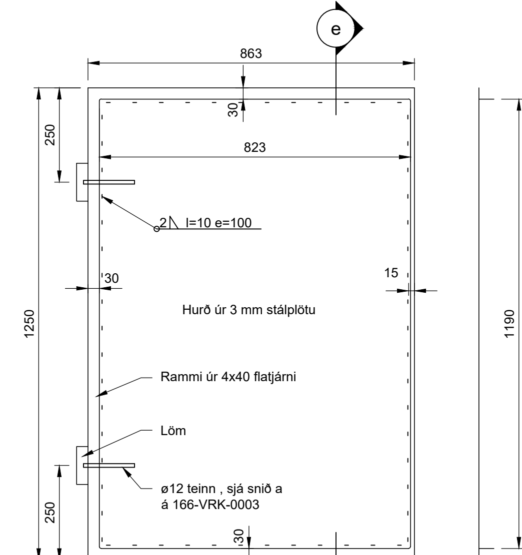
HURDIR 1:10
