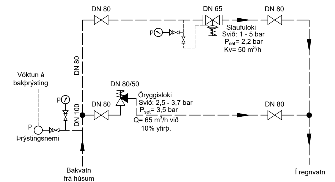
KERFISMYND
