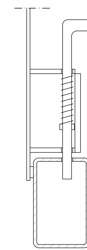
b SNIÐ 1:2
