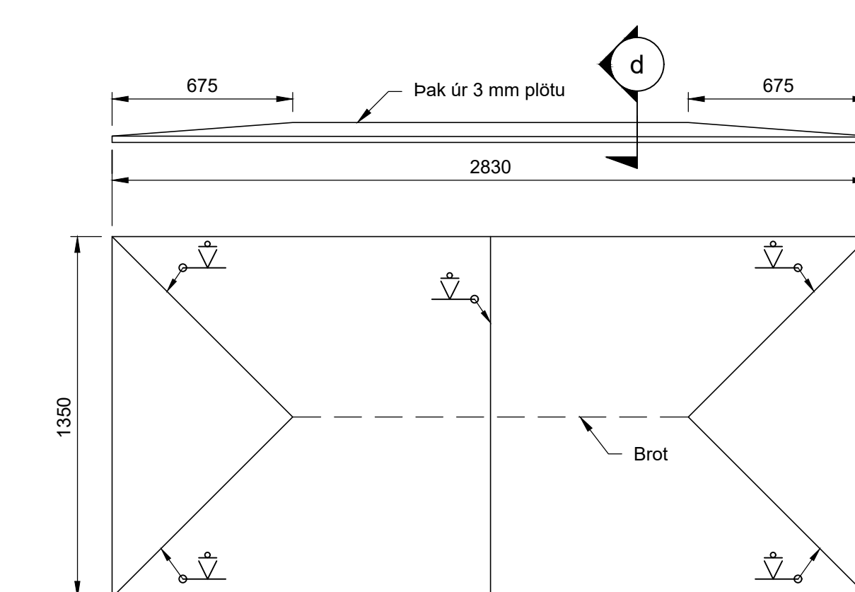
P ÞAK 1:20
