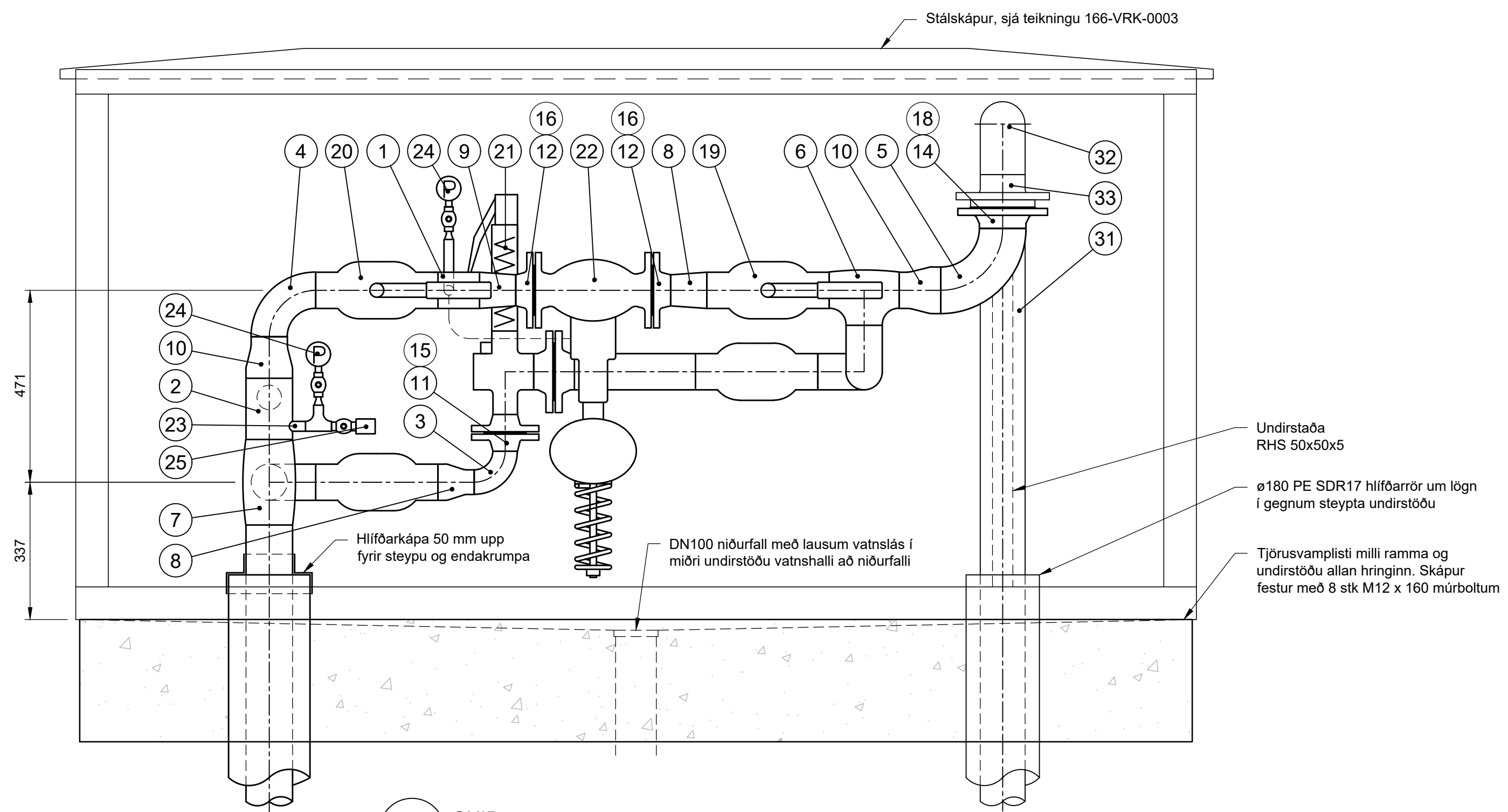
a SNIÐ 1:10
