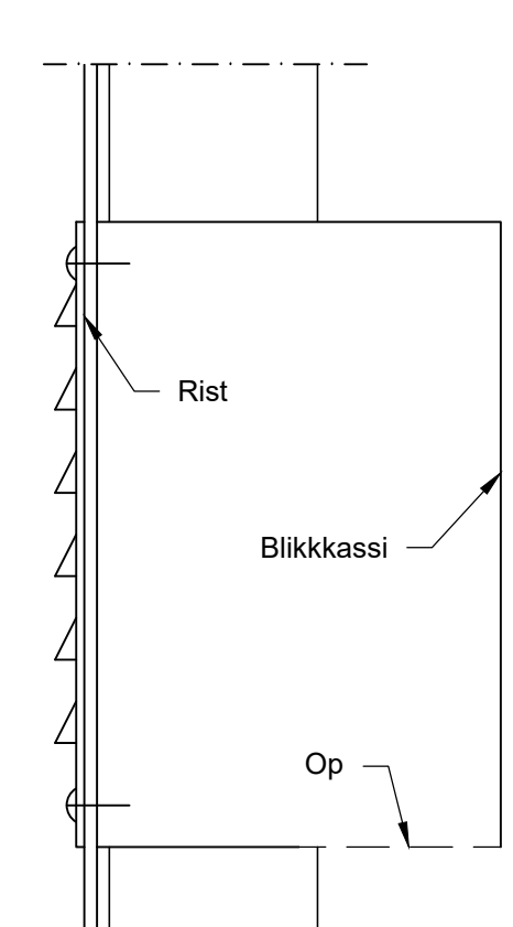
L LOFTTÚÐA 1:2
