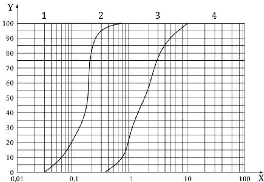
Mynd 2: Kornakúrfa sandlags 0,02/10mm, skilgreining skv. ÍST EN 13941-2:2019, X-ás gefin upp í mm og y-ás gefin upp í hlutfalli [%] af heildarþyngd.
