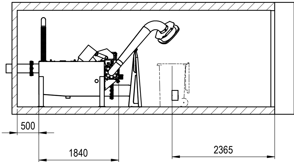
A-A ( 1:50 )
