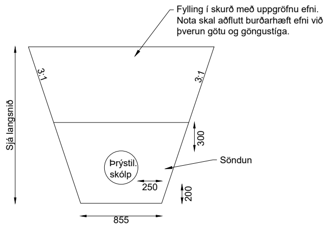
A KENNISNIÐ A 1:20
