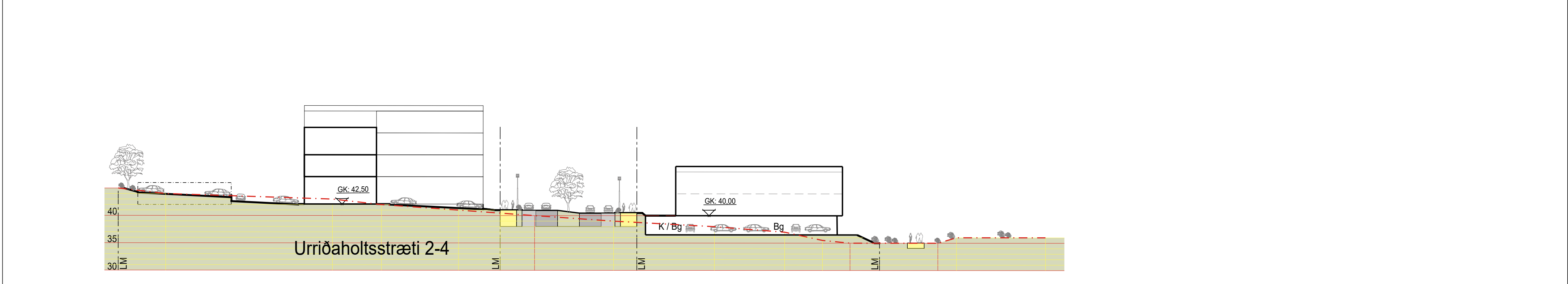
Snið A-A Urriðaholtsstræti Göngustígur - útivistarsvæði
