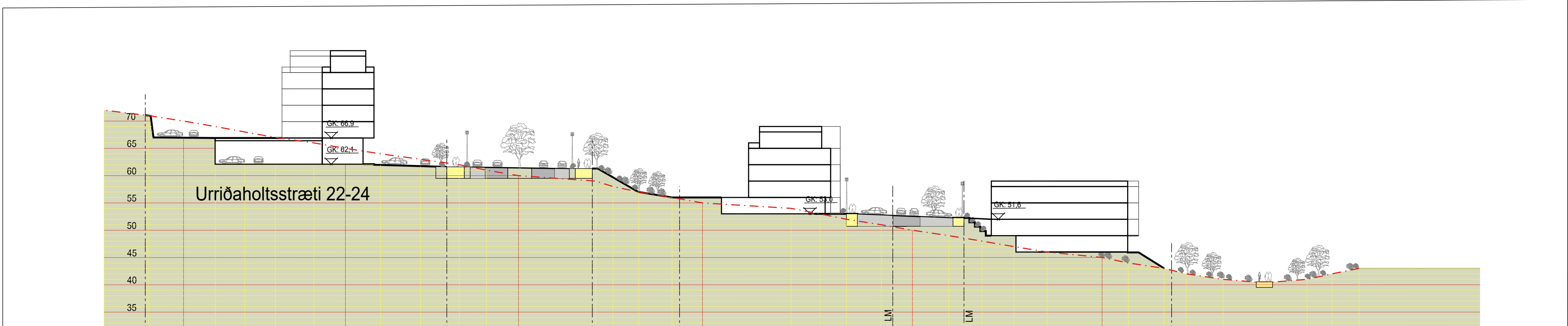
Snið E-E Urriðaholtsstræti Göngustígur - útivistarsvæði
