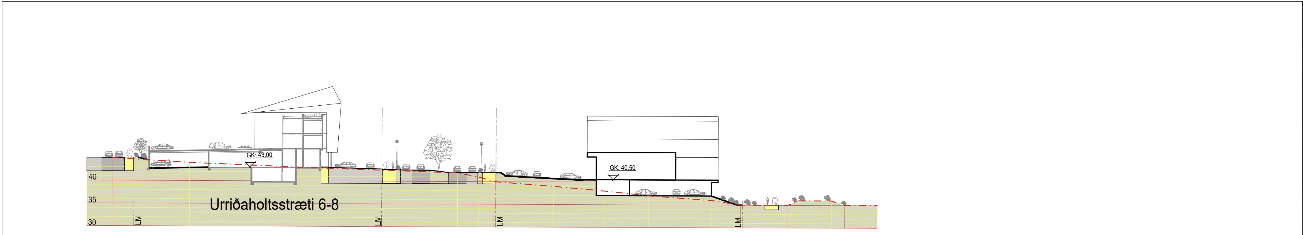
Snið B-B Urriðaholtsstræti Göngustígur - útivistarsvæði
