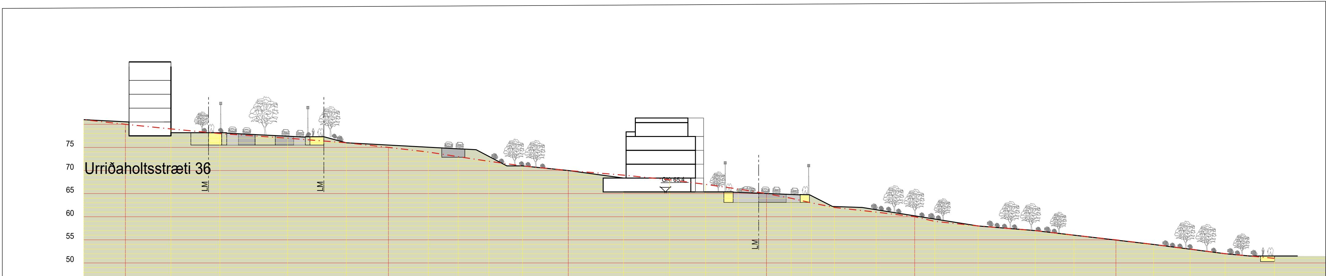
Snið F-F Urriðaholtsstræti Útivistarsvæði
