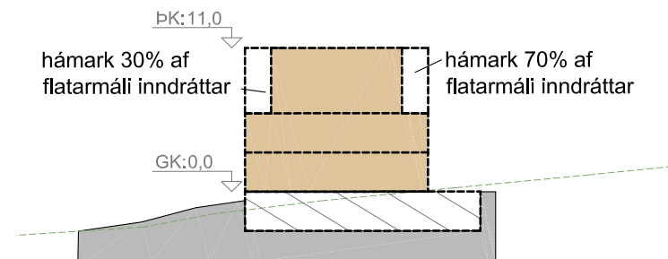
Sneiðing B-B
