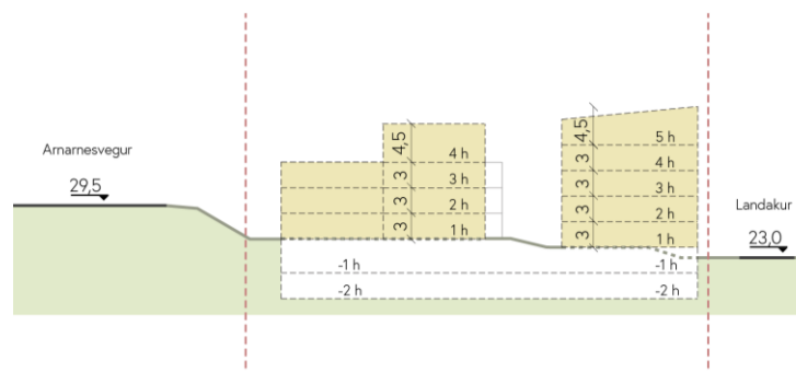
Snið BB
