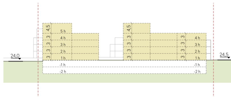
Snið AA
