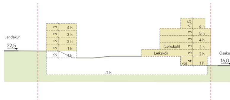
Snið AA
