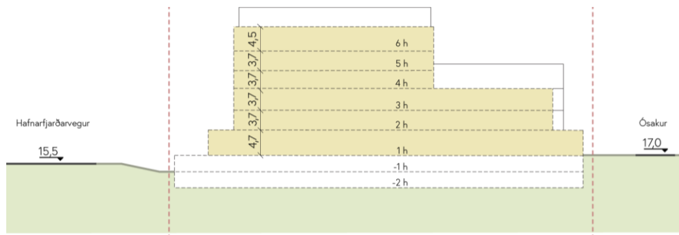
Snið BB
