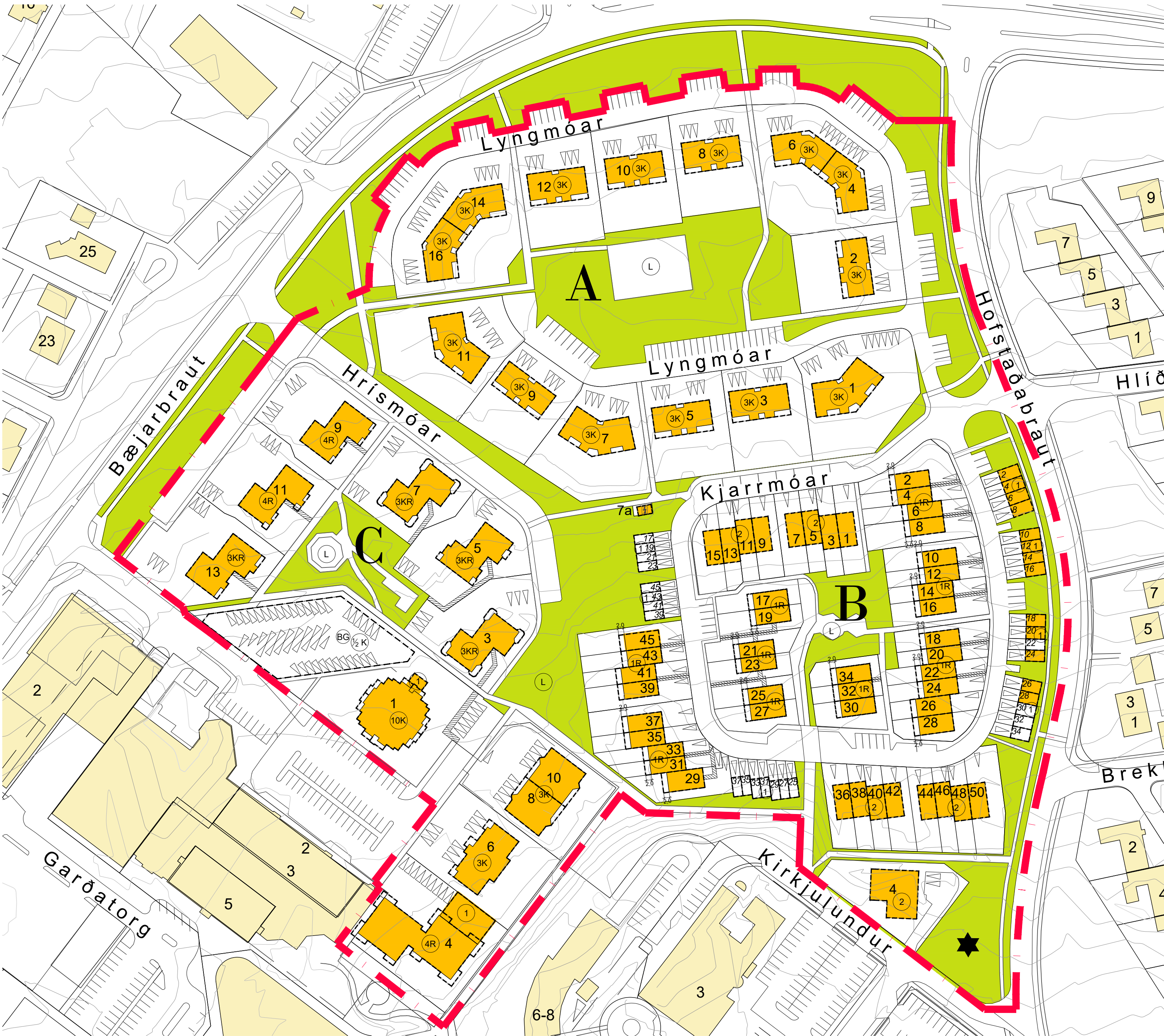
DEILISKIPULAGSUPPDRÁTTUR MKV 1 : 1000
