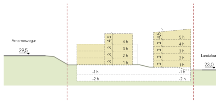
Snið BB
