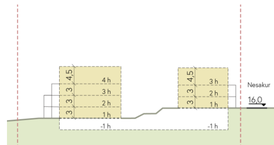
Snið AA
