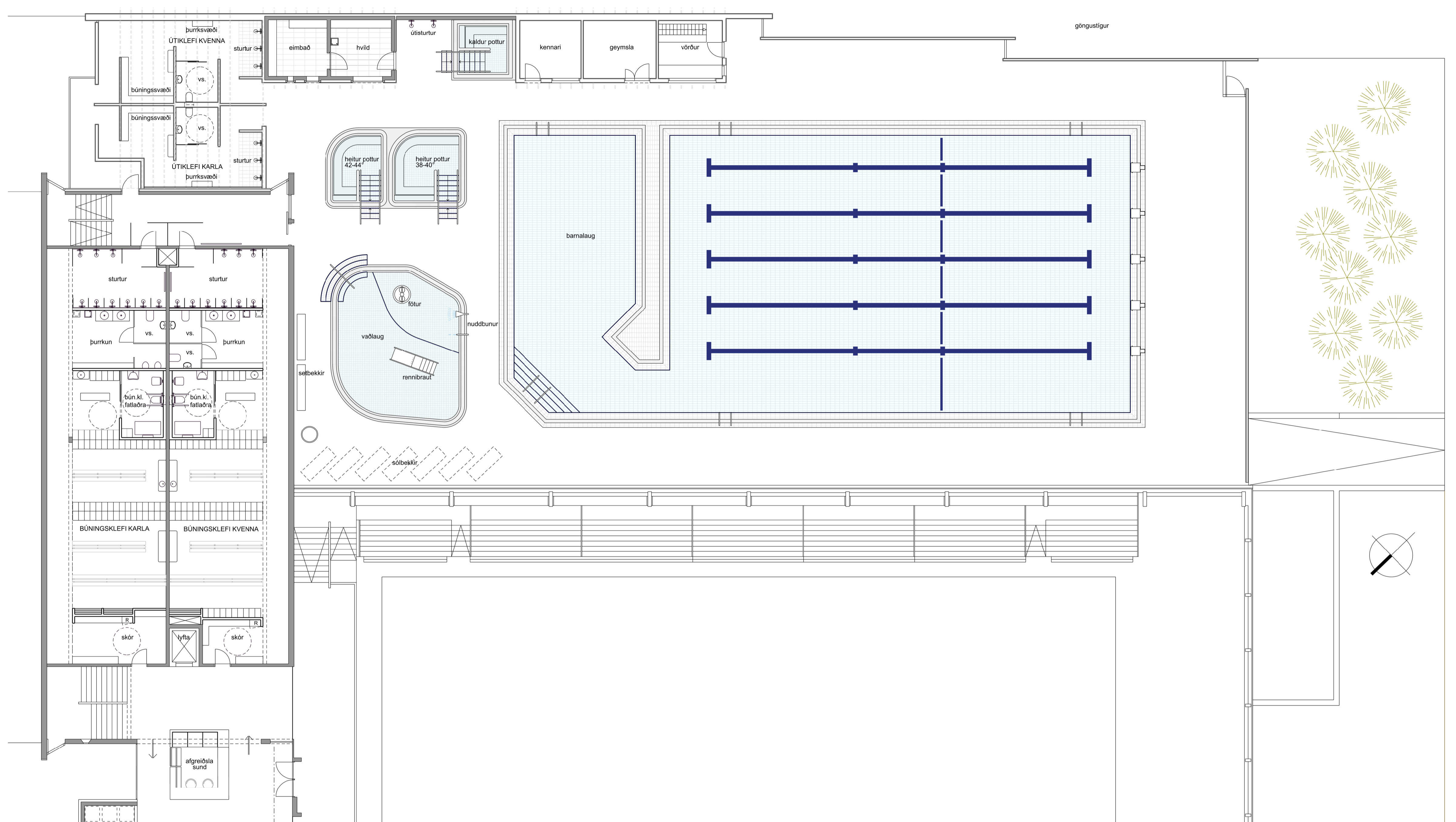
GRUNNMYND 1. HÆÐ - KLEFAR OG SUNDLAUGARSVÆÐI
