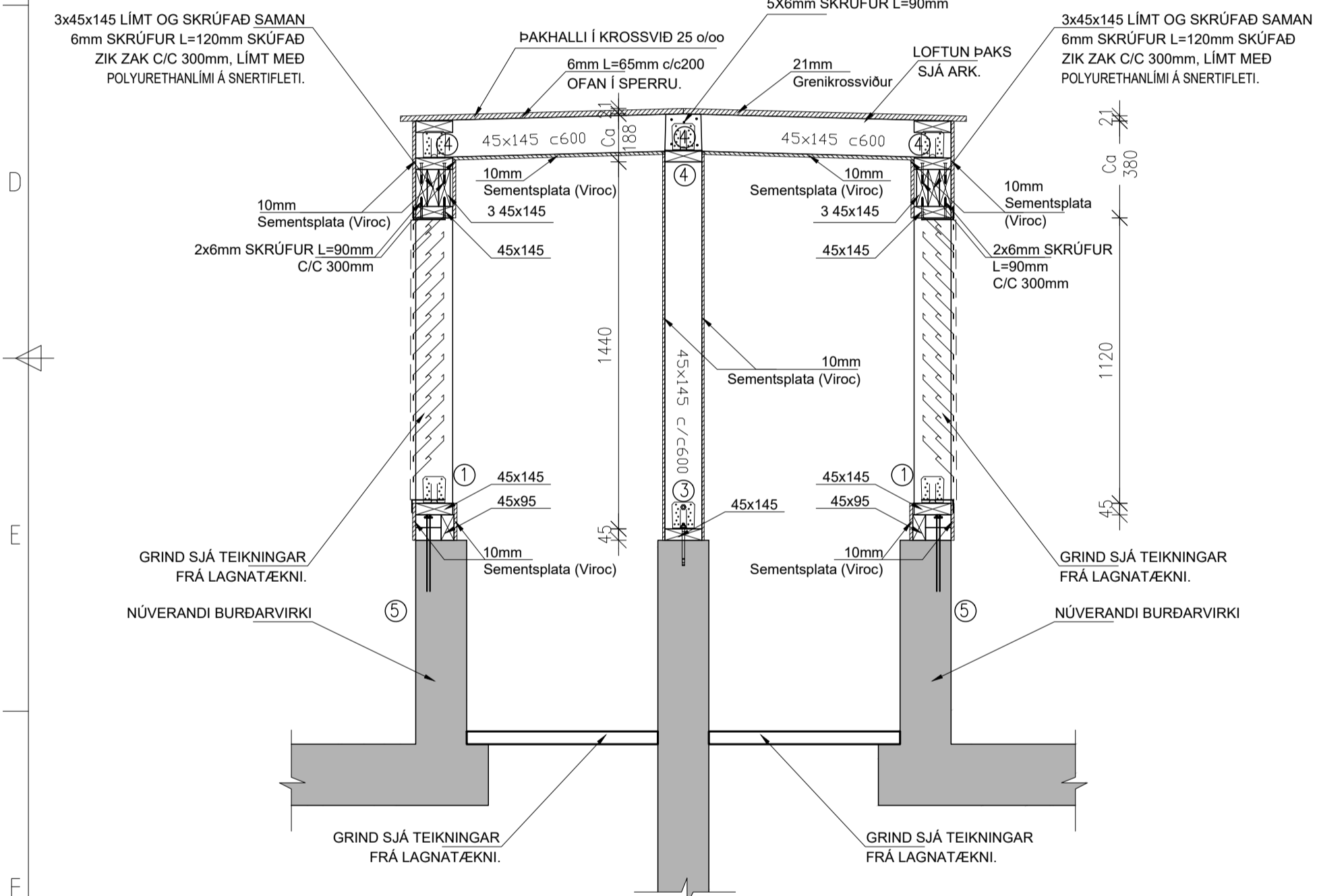
A SNID M. 1: 20
