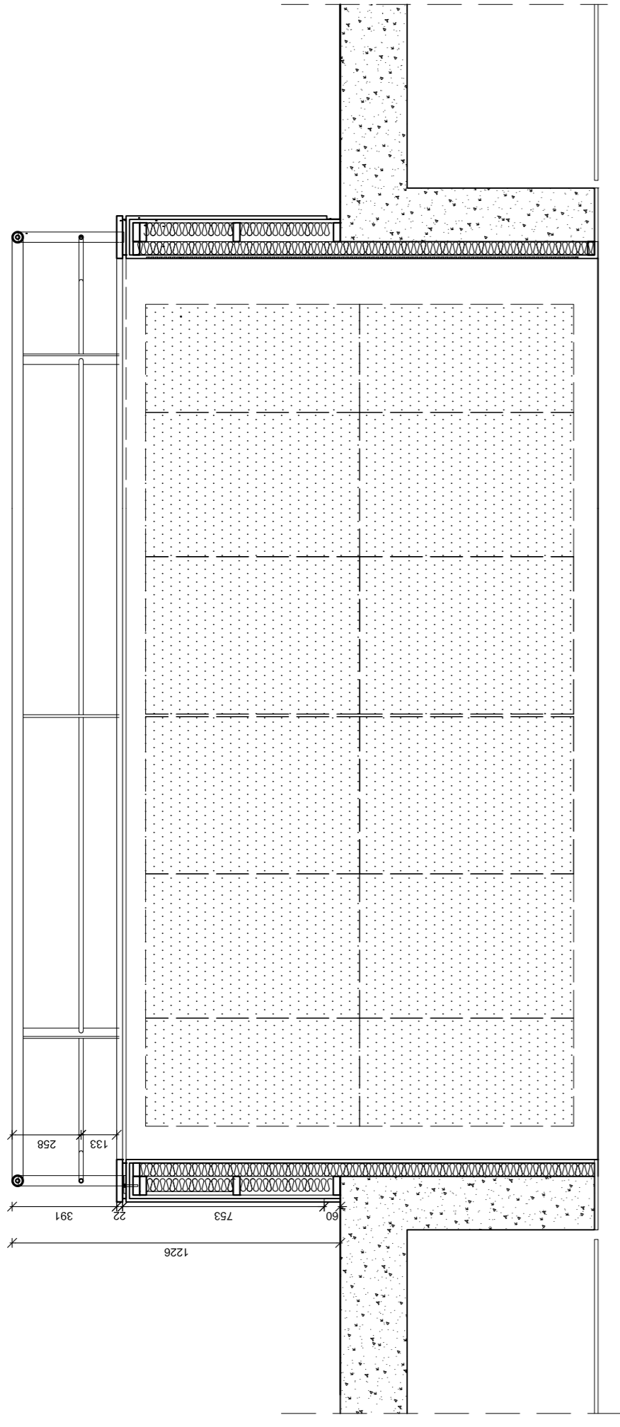
HA-3 Ásýnd og snið AA m.kv. 1:20
