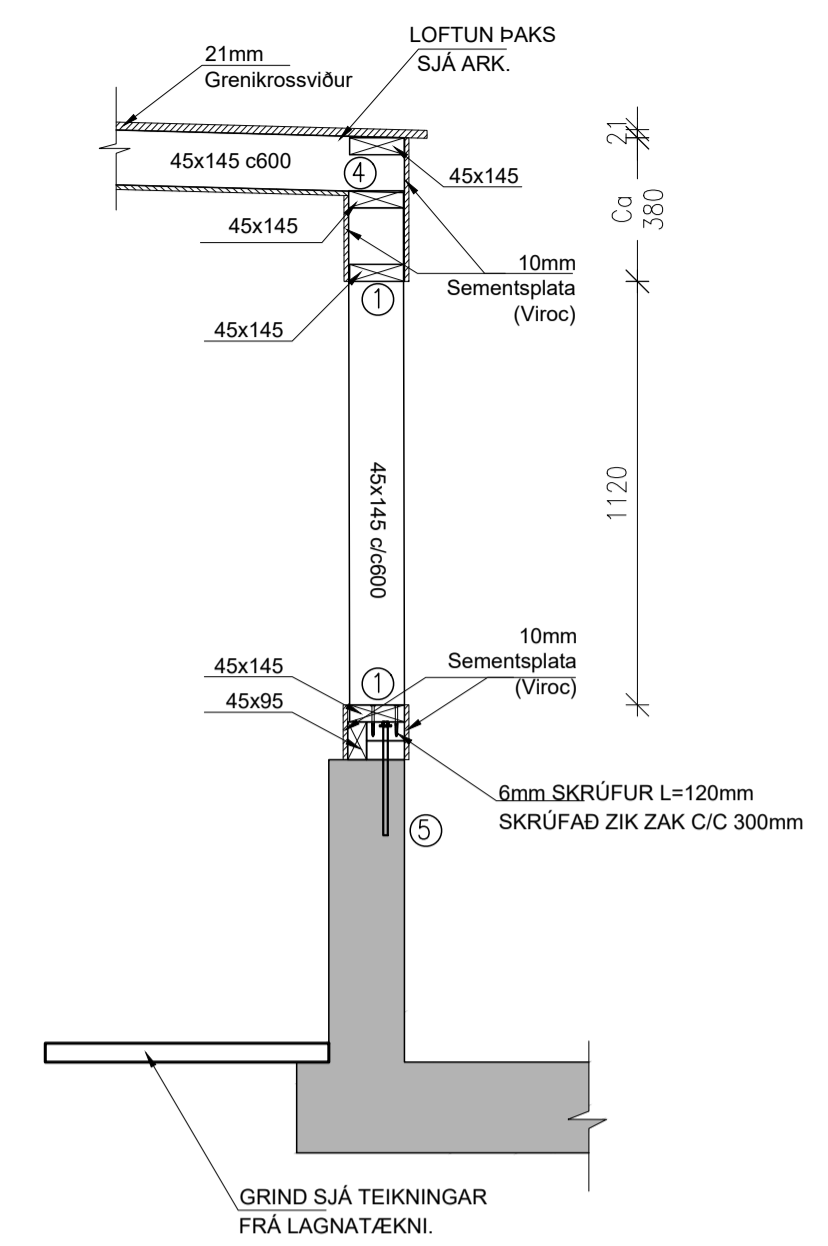
C SNID M. 1: 20
