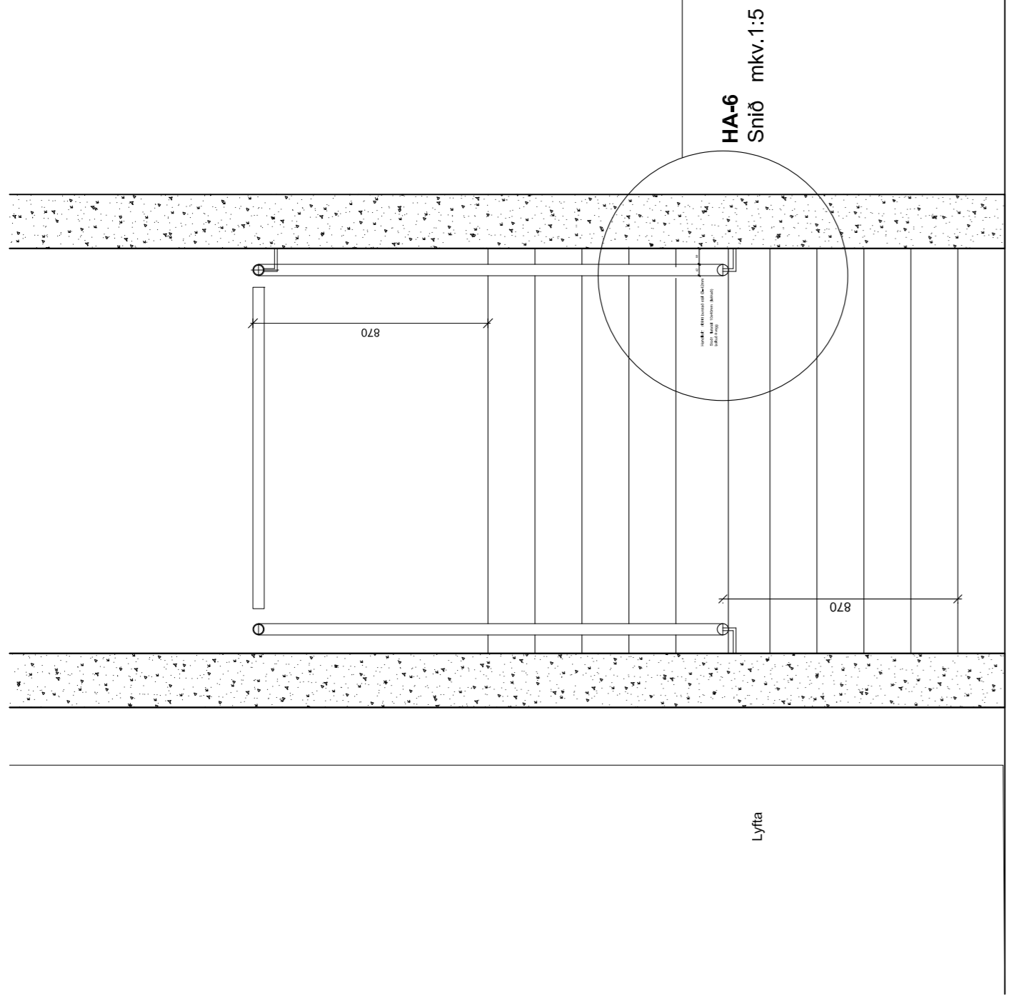
HA-6 Ásýnd á stíga m.kv.1.20
