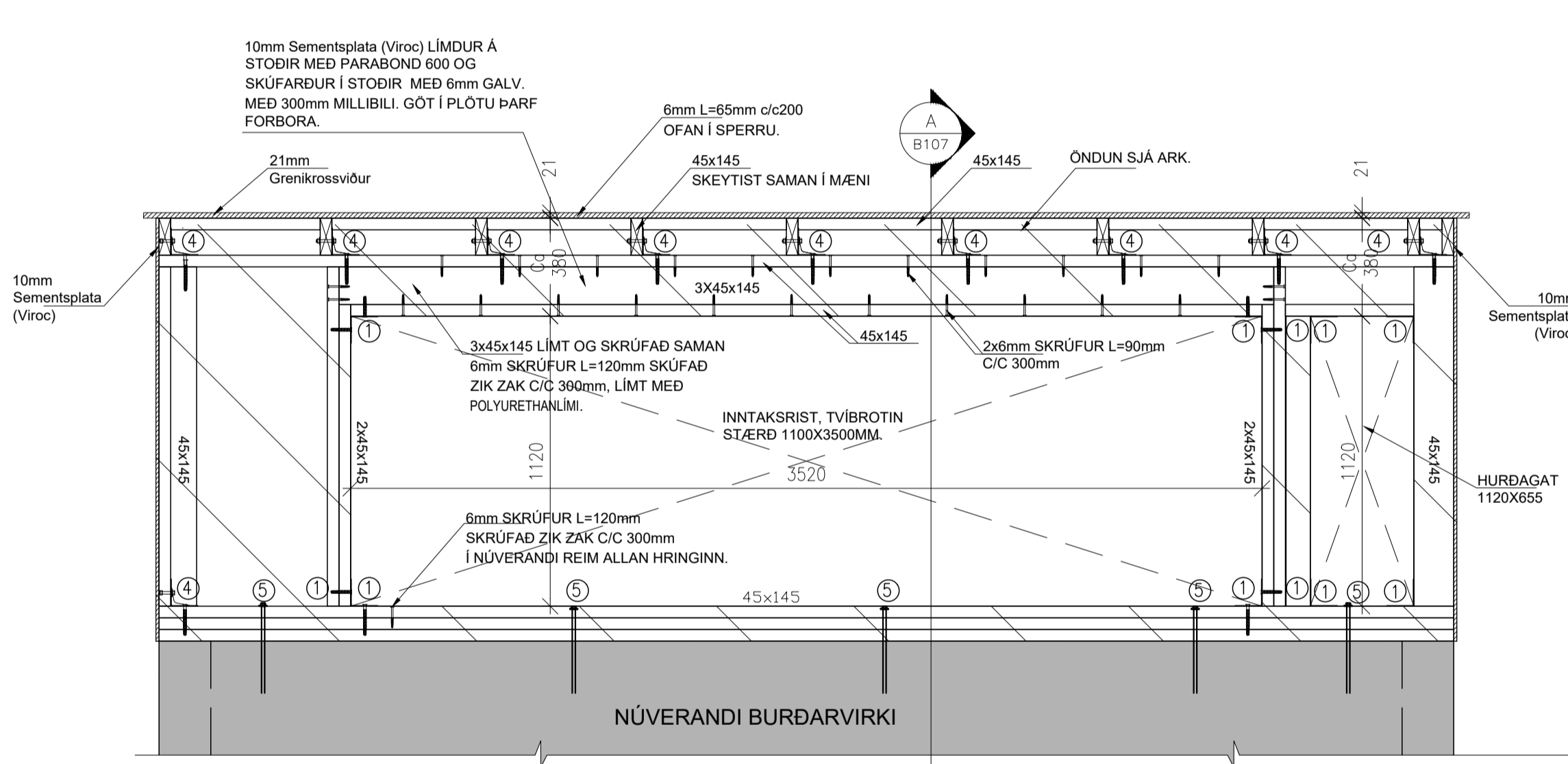
GRIND 1 M 1:20
