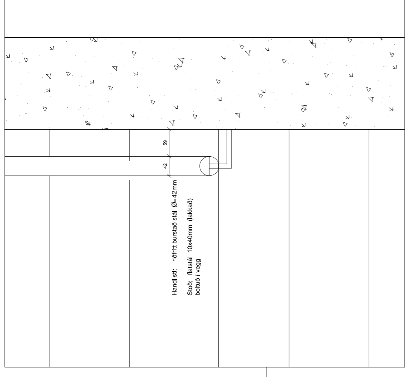
HA-6 Snúð m.kv.1.5
