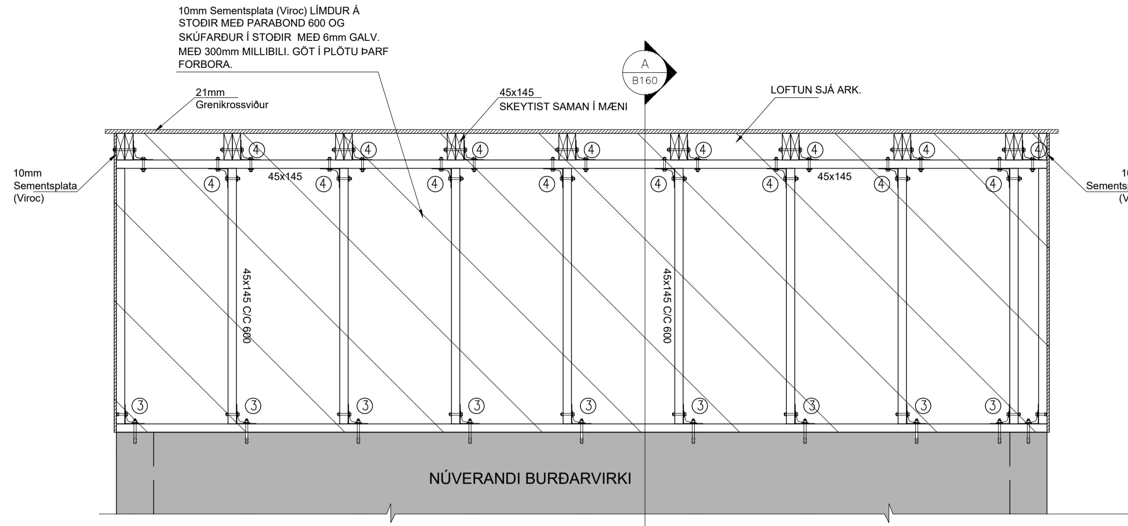
B SNID M. 1: 20
