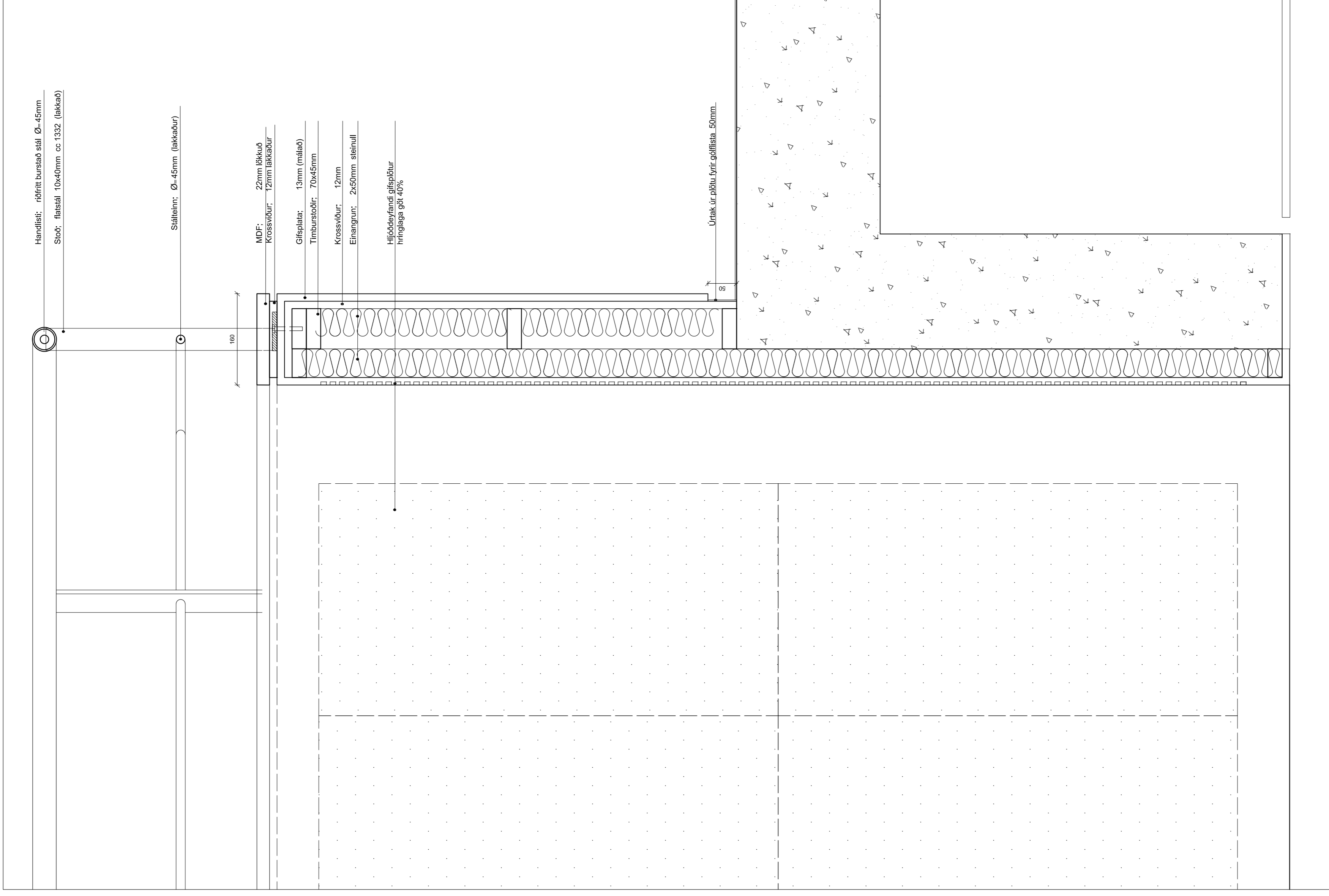
Skurður í vegg m.kv. 1:5
