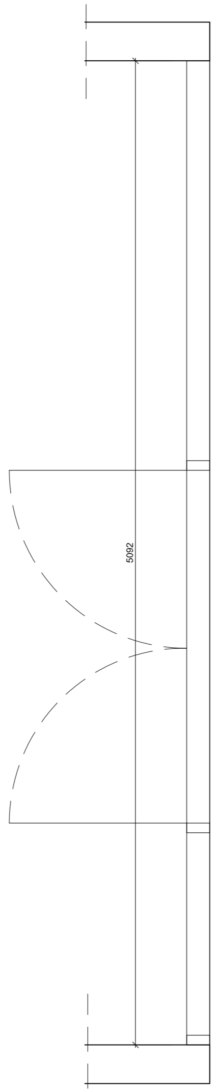
IH-20 1 stik Innihurð og gluggi úr áli. (anddyri) Ath Öryggisgler í glugga, paníkklá og bursit undir hurðum
