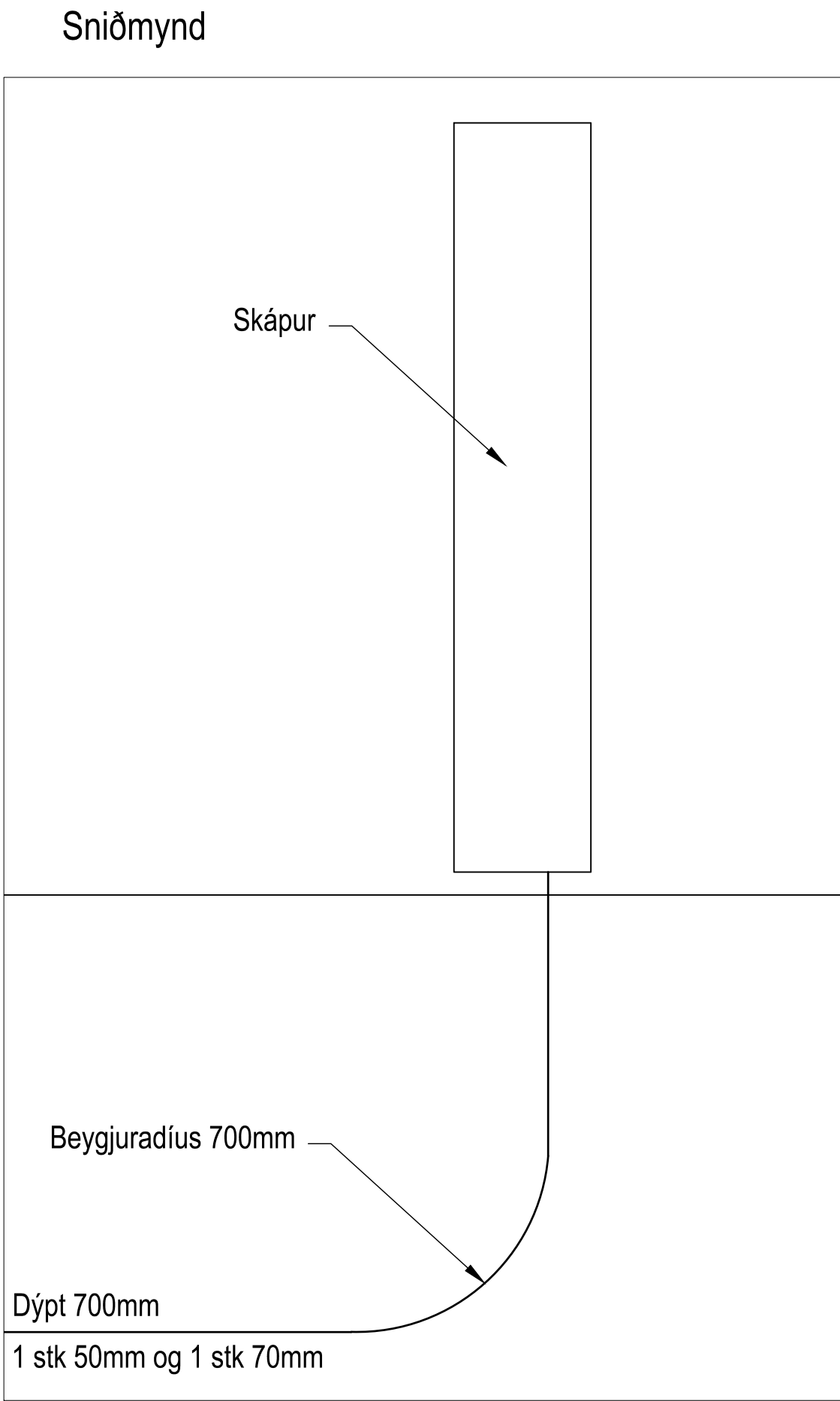
Sniðmynd
