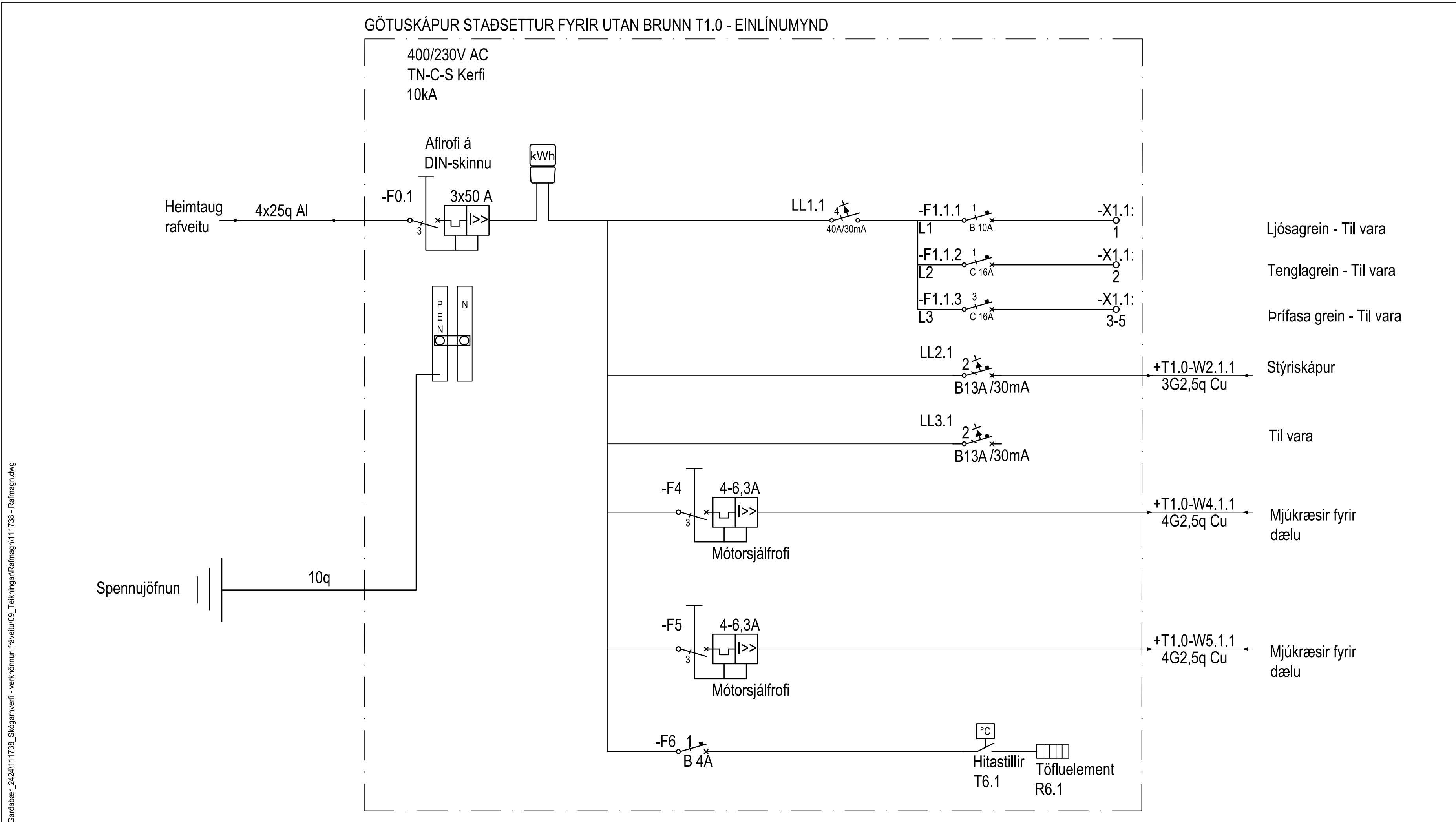
Einlínumynd
